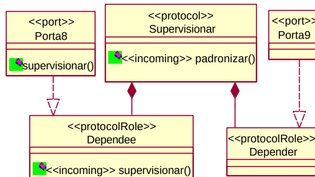
Figura A.30 - Protocolo Supervisor representando uma dependência de tarefa entre as cápsulas Agência Intermediária e Coordenação.
