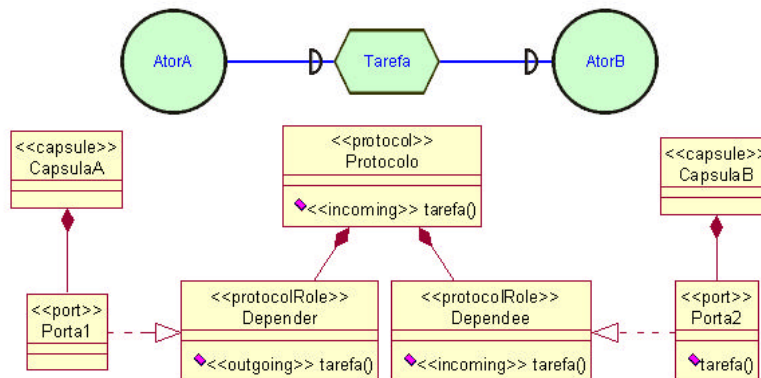
Figura 5.15 - Mapeando uma dependência de tarefa para UML
