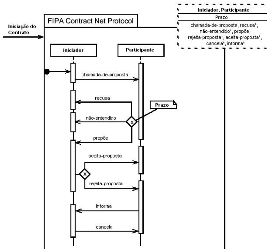
Figura 3.3 - Um Protocolo de Interação de Agente genérico expressado como um pacote modelo
