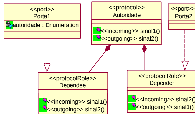
Figura A.37 - Protocolo Autoridade representando uma dependência de meta-soft entre as cápsulas Negociador e Executivo
