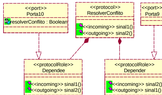
Figura A.40 - Protocolo ResolverConflito representando uma dependência de meta entre as cápsulas Ponderador e Controlador
