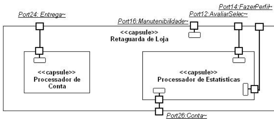
Figura 6.10 - Refinamento da Cápsula Retaguarda de Loja
