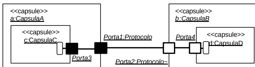
Figura 4.3 - Um diagrama de colaboração de Cápsulas
