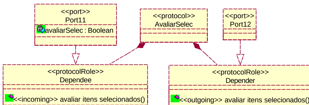
Figura B.16 - Protocolo AvaliarSelec representando uma dependência de meta entre as cápsulas Retaguarda de Loja e Frente de Loja
