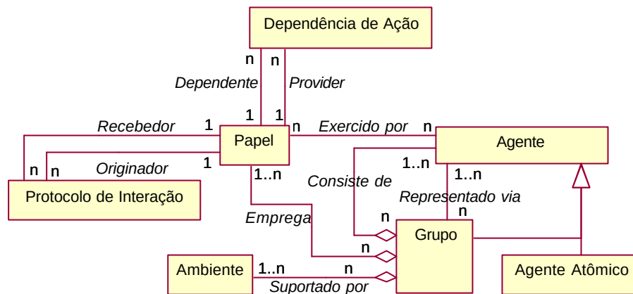
Figura 3.6 - Ontologia Consolidada
