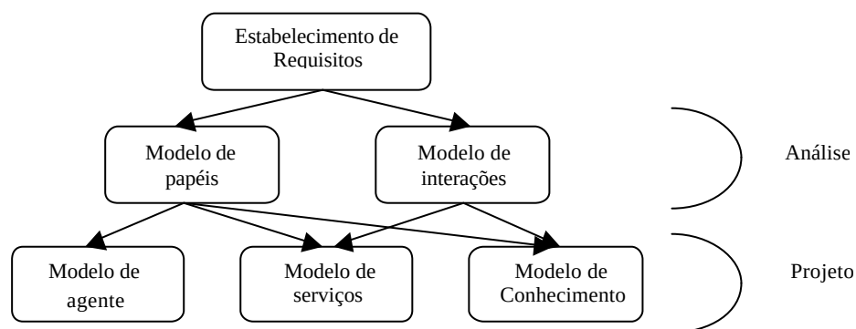
Figura 3.2 - Relacionamentos entre os modelos Gaia
