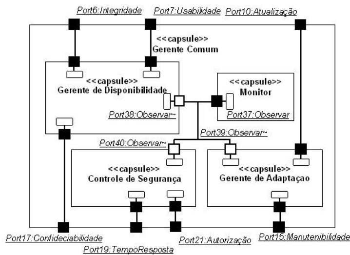
Figura 6.8 - Refinamento da Cápsula Gerente Comum
