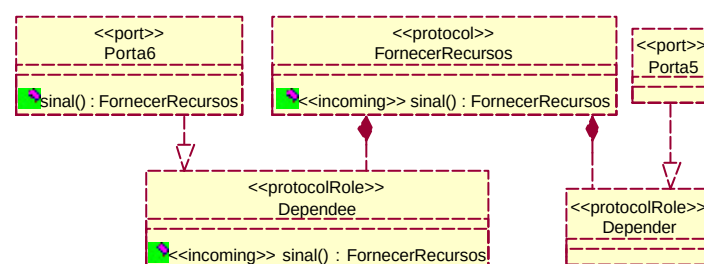
Figura A.51 - Protocolo FornecerRecursos representando uma dependência de recurso entre as cápsulas Tomador de Controle e Agência 3
