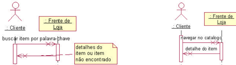
Figura 6.14 - Diagrama de sequência para o contexto Pesquisar Item. (a) Buscar item por palavra-chave. (b) Navegar no catálogo da Loja de Mídia
