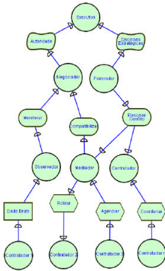
Figura 5.8 - Contratação Hierárquica (Hierarchical Contracting)
