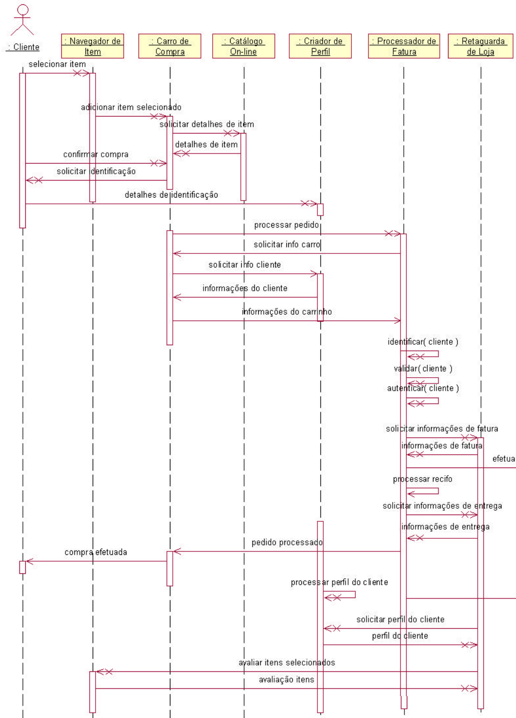
Figura 6.15 - Diagrama de sequência refinando a Frente de Loja para o contexto Fazer Pedido
