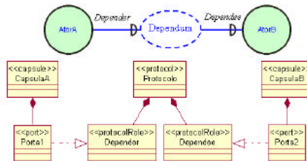
Figura 5.11 - Mapeando uma dependência entre atores para UML
