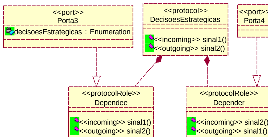
Figura A.38 - Protocolo DecisoeseStrategicas representando uma dependência de meta-soft entre as cápsulas Ponderador e Executivo
