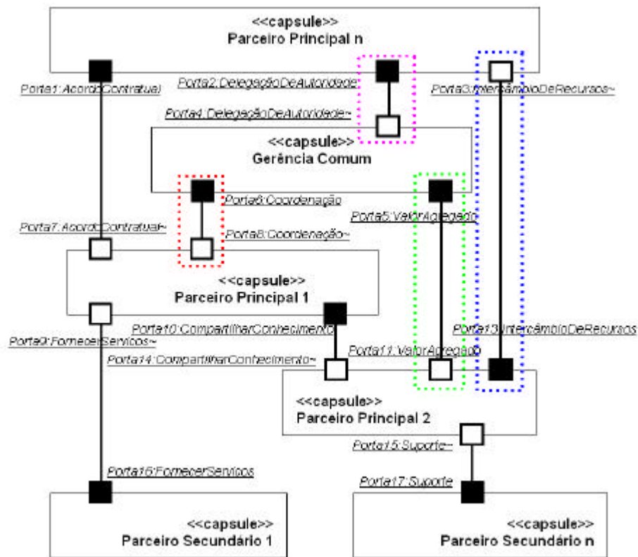
Figura 5.16 - Estilo União Estratégica em UML-RT
