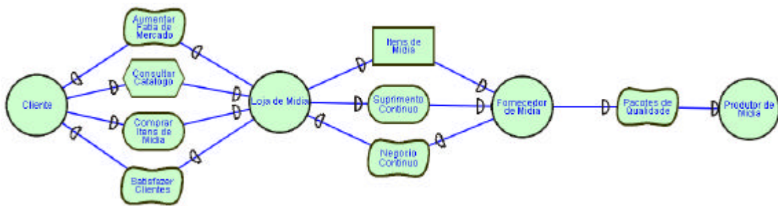
Figura 6.1 - Modelo i* de Dependência Estratégica da Loja de Mídia
