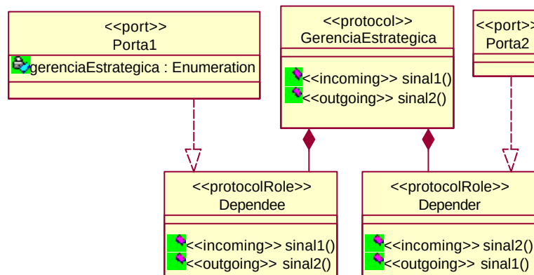
Figura A.26 - Protocolo GerênciaEstratégica representando uma dependência de meta-soft entre as cápsulas Agência Intermediária e Cúpsula.
