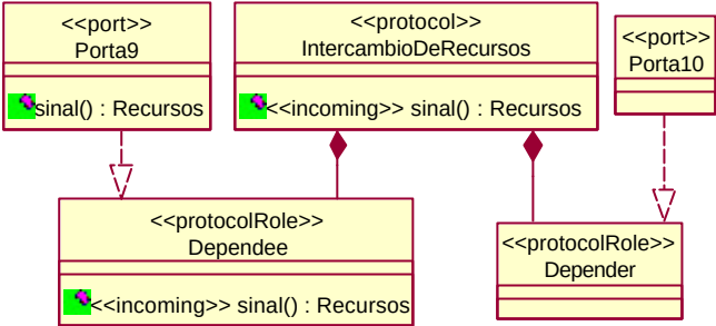
Figura A.64 - Protocolo IntercambioDeRecursos representando uma dependência de recurso entre as cápsulas Agência 3 e Agência n
