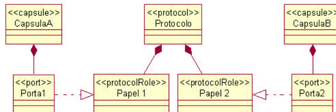
Figura 4.2 - Um diagrama de classes de Cápsula detalhado
