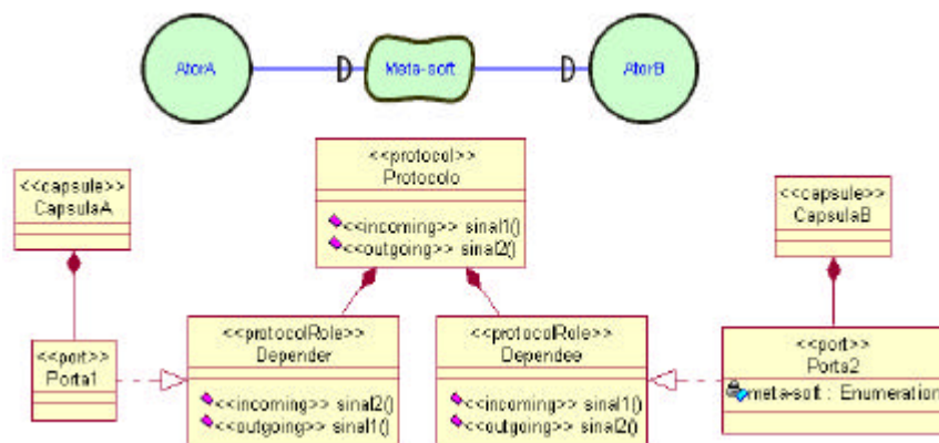
Figura 5.13 - Mapeando uma dependência de meta-soft para UML
