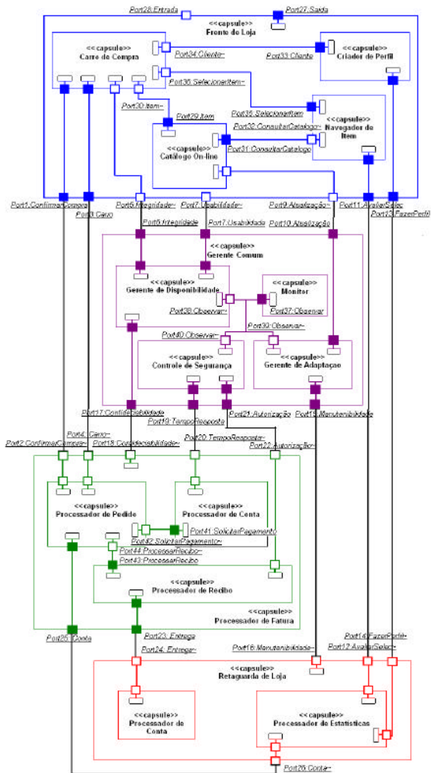
Figura 6.11 - O refinamento da arquitetura do sistema Medi@
