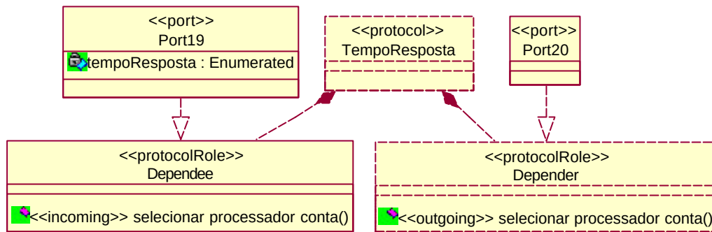
Figura B.18 - Protocolo TempoResposta representando uma dependência de meta-soft entre as cápsulas Processador de Fatura e Gerente Comum
