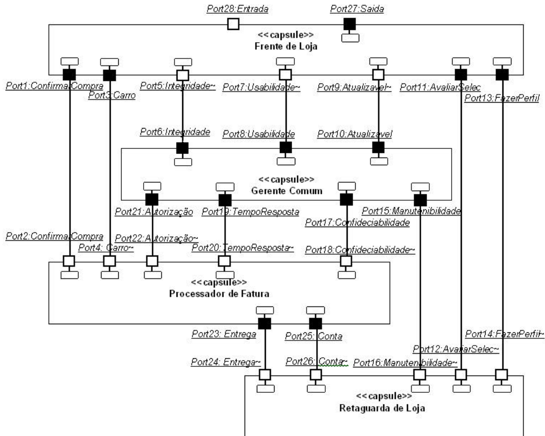
Figura 6.6 - A arquitetura União Estratégica do sistema Media@
