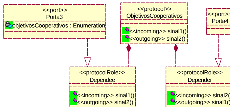
Figura A.45 - Protocolo ObjetivosCorporativos representando uma dependência de meta-soft entre as cápsulas Colaborador 3 e Colaborador 1
