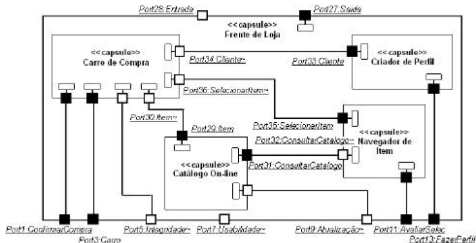
Figura 6.7 - Refinamento da cápsula Frente de Loja
