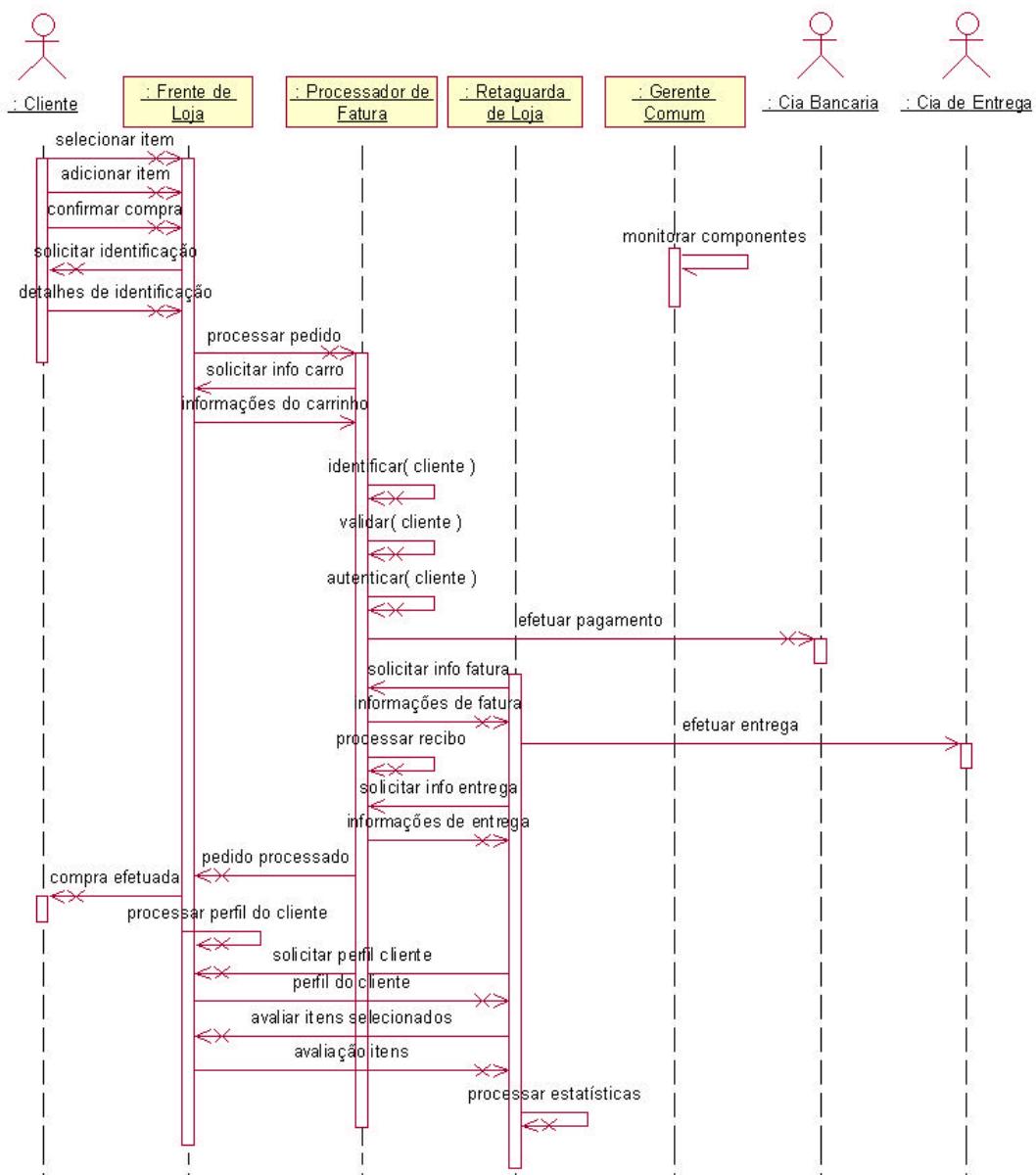
Figura 6.12 - Diagrama de seqüência para o contexto Fazer Pedido
