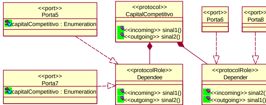
Figura A.44 - Protocolo CapitalCompetitivo representando uma dependência de meta-soft entre as cápsulas Colaborador 1, Colaborador 2, Colaborador 3 e Colaborador n
