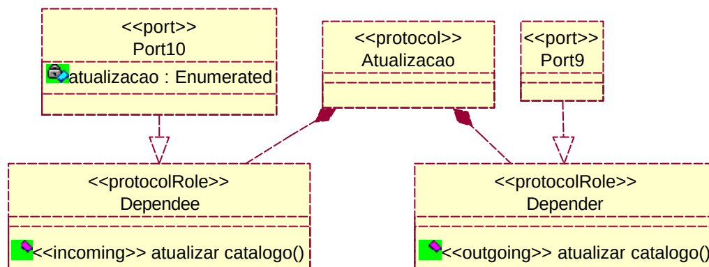
Figura B.13 - Protocolo Atualização representando uma dependência de meta-soft entre as cápsulas Frente de Loja e Gerente Comum
