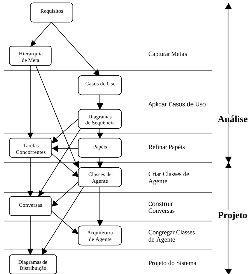
Figura 3.8 - Metodologia MaSE
