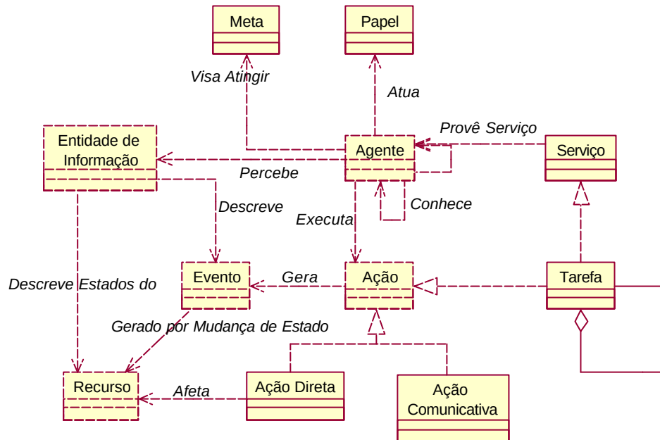
Figura 3.7 - Conceitos MESSAGE
