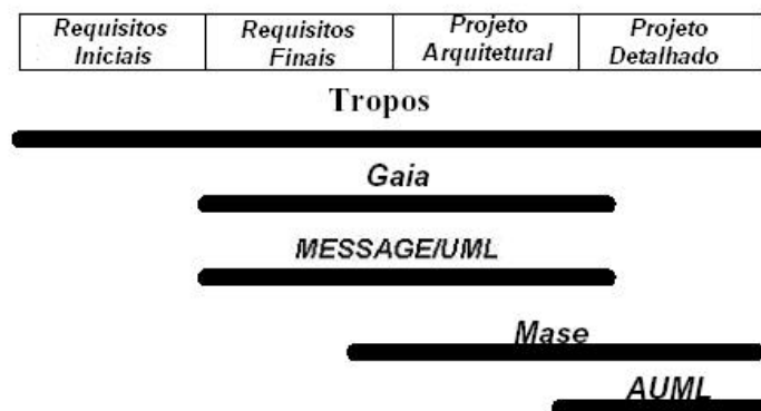
Figura 3.9 - Cobertura das fases de desenvolvimento do software
