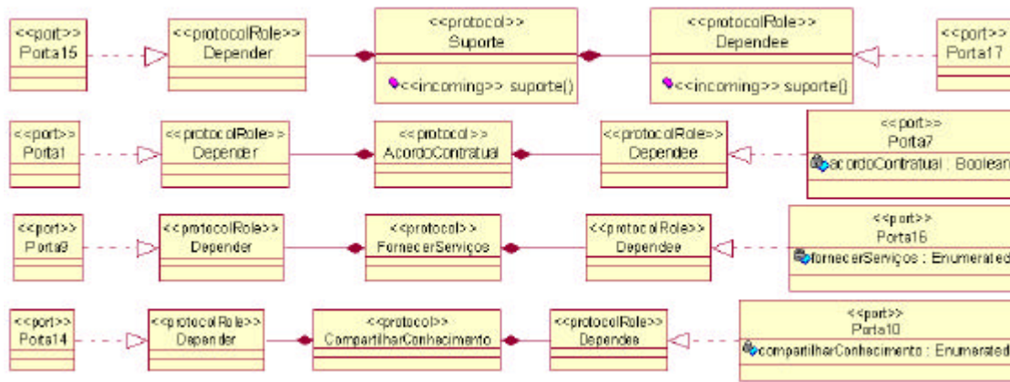
Figura 5.21 - Protocolos e portas que representam as demais dependências do estilo União Estratégica
